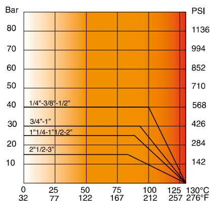
Diagramma pressione/temperatura (prova eseguita con acqua)
