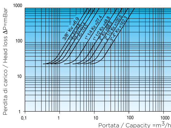
Diagramma perdite di carico (prova eseguita con acqua)
